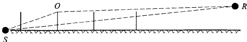
Figura 2.5.i: Diferența traiectoriei pentru a doua reflexie
