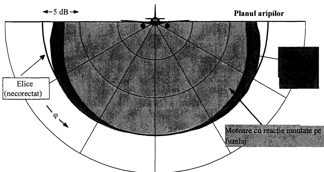
Figura 2.7.n: Direcționalitatea laterală a efectelor amplasării
