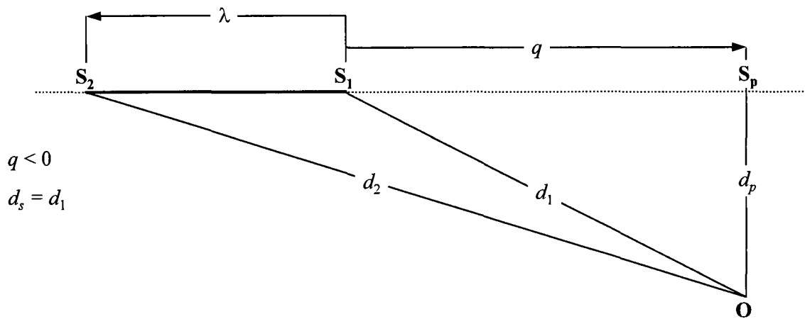
Figura 2.7.j: Geometria segmentului traiectului de zbor pentru poziția observatorului în spatele segmentului
