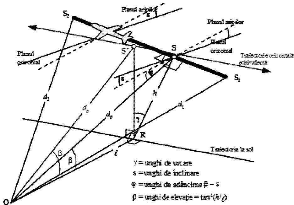
Figura 2.7.p : Observatorul în dreptul segmentului
